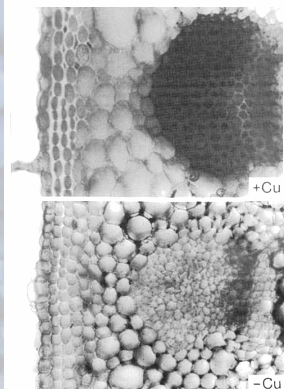
Arriba, sección de tallo de girasol con buen aporte de cobre (50mg Cu/l) con paredes gruesas y lignificadas y abajo, una sección de tallo de girasol deficiente en cobre con paredes celulares delgadas y sin lignificar. (Rahimi & Bussler, 1974.)
